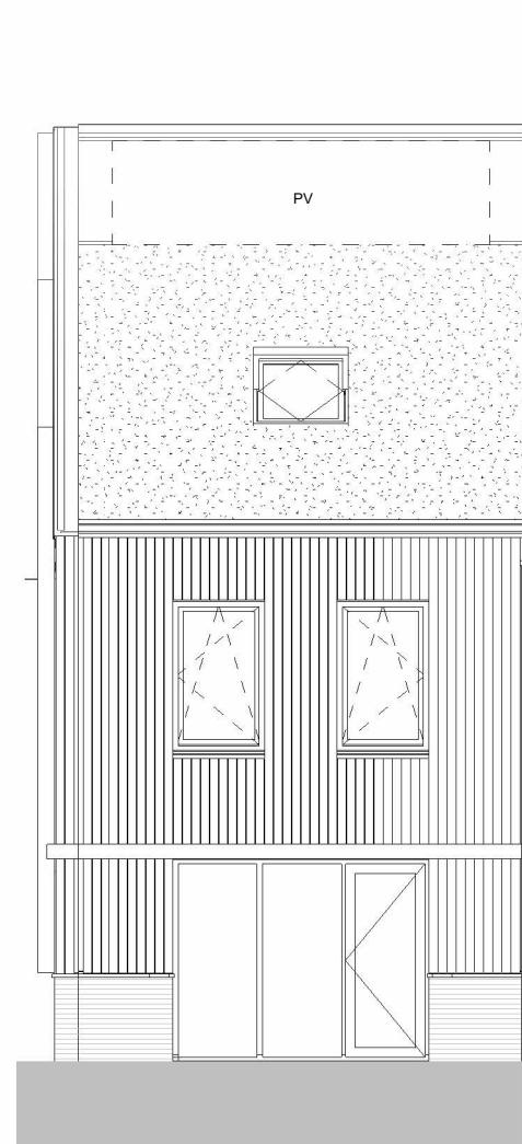
achtergevel
