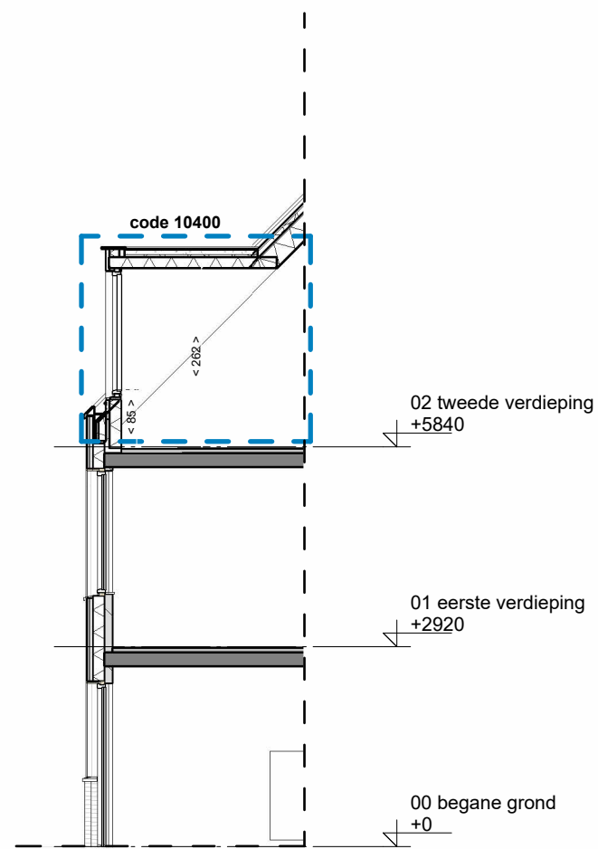
doorsnede
