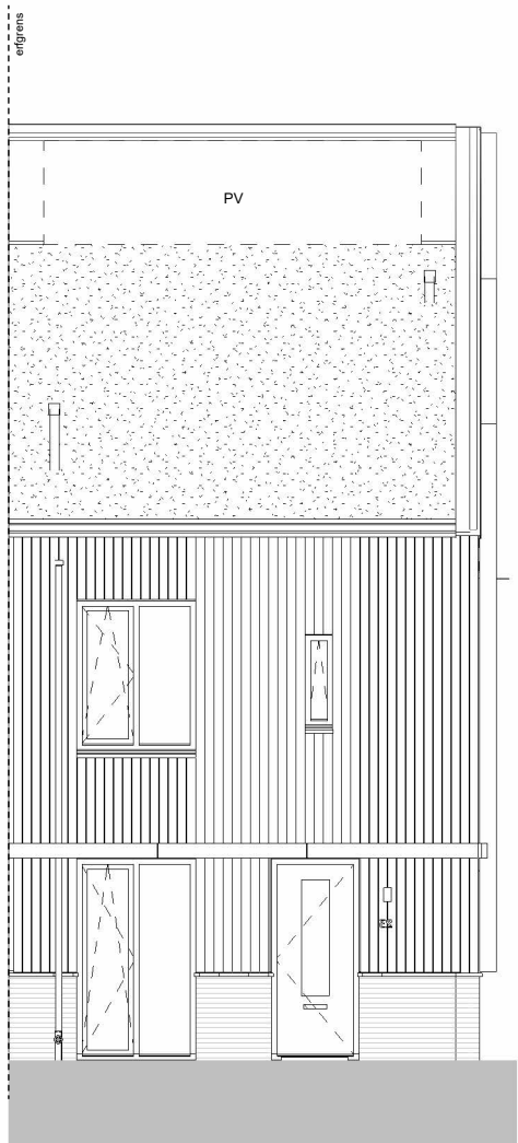
voorgevel
